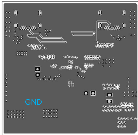
Middle Layer 2
