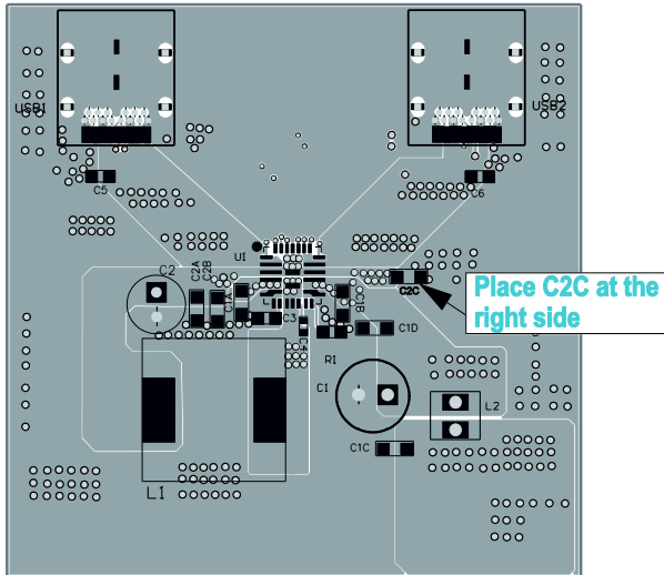
Top Layer
