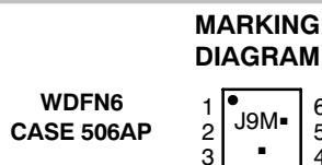
P-CHANNEL MOSFET
