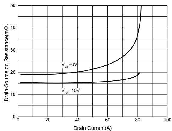
Fig.4 RDS(ON)-Id
