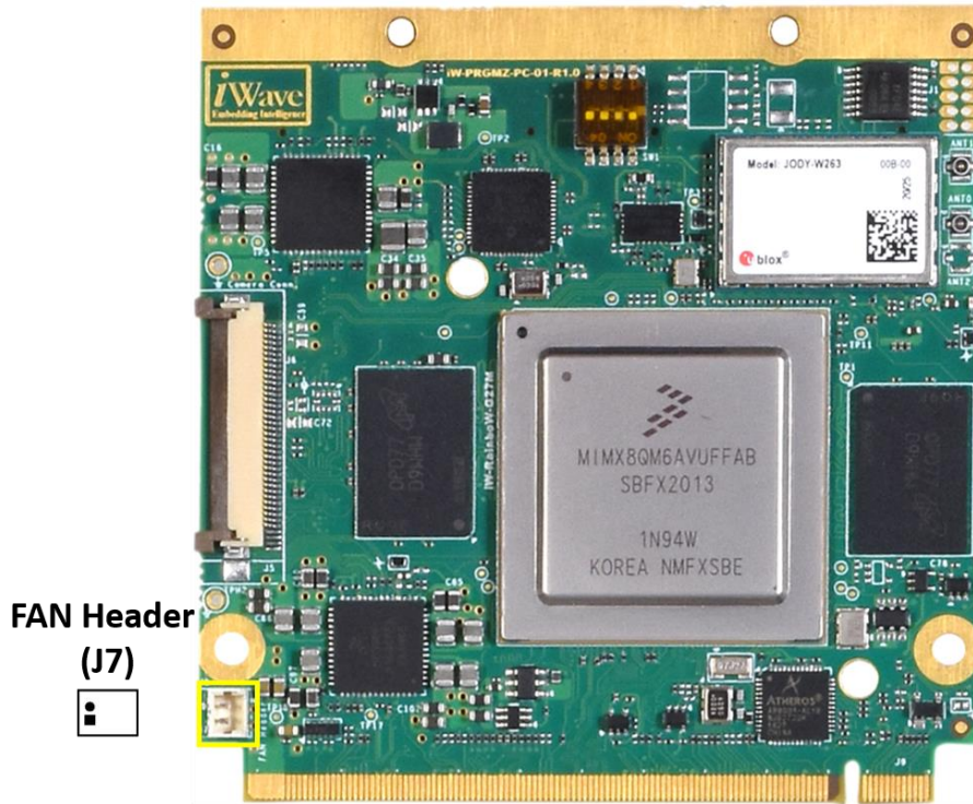
Figure 10: FAN Header
