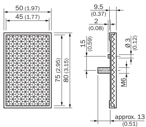
尺寸图 (尺寸单位: mm)
