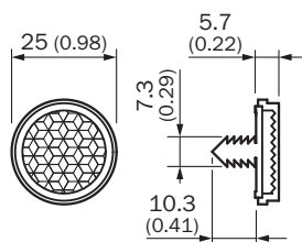
尺寸图 (尺寸单位: mm)
