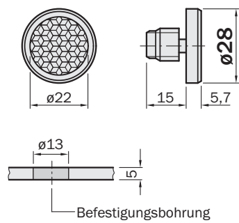
尺寸图 (尺寸单位: mm)
