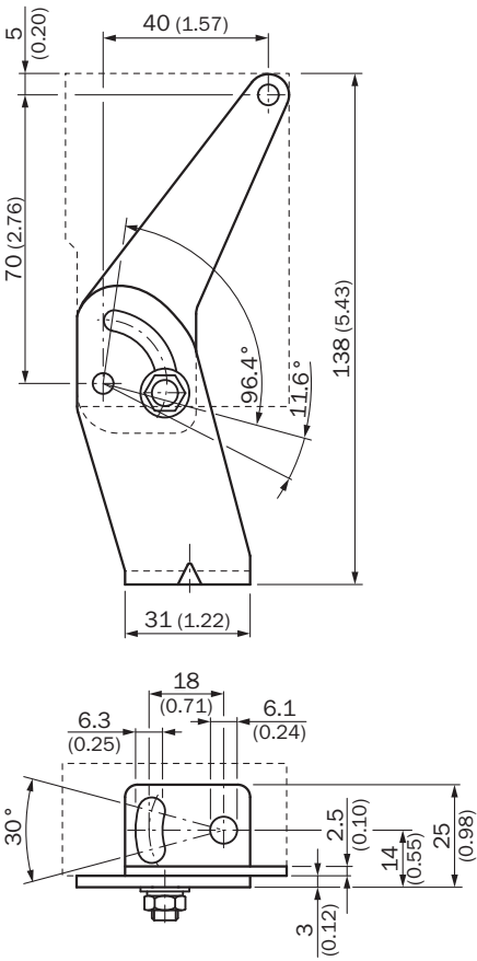
尺寸图 (尺寸单位: mm)
