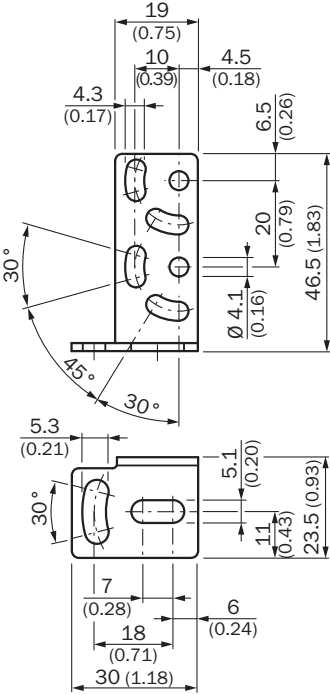
尺寸图 (尺寸单位: mm)
