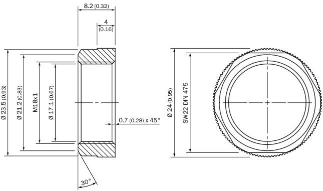
尺寸图 (尺寸单位: mm)
