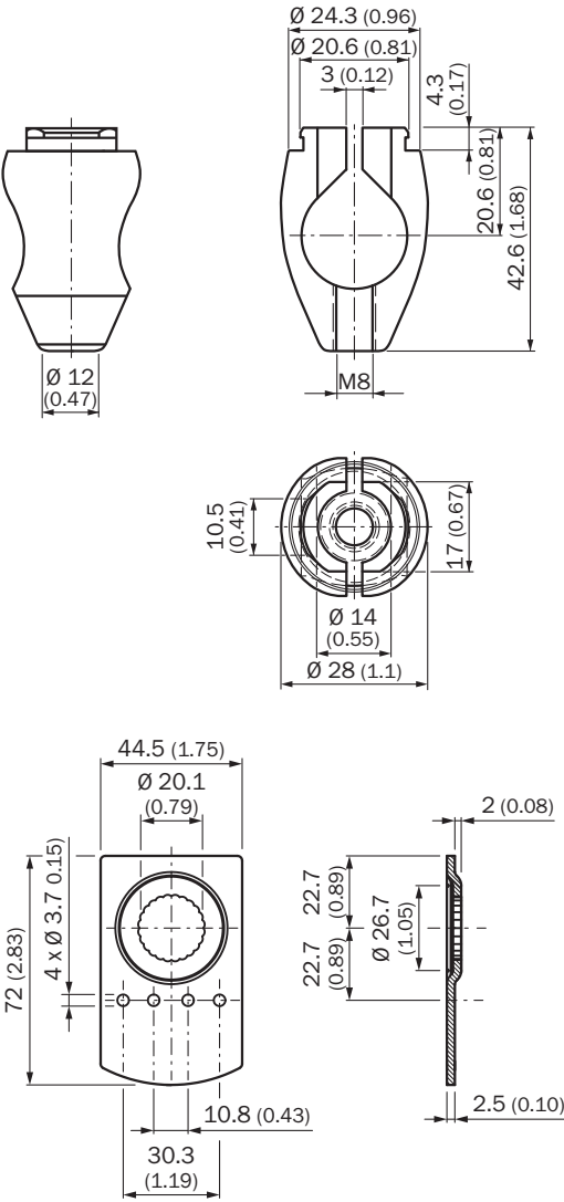
尺寸图 (尺寸单位: mm)
