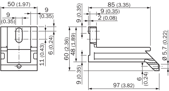
尺寸图 (尺寸单位: mm)
