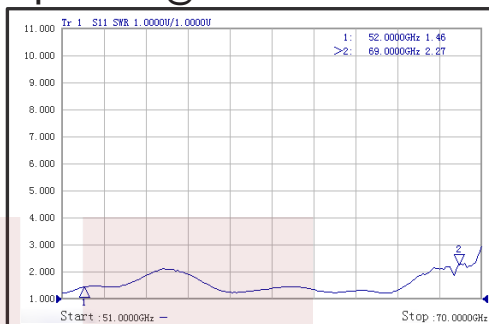
Input VSWR@+25°C
