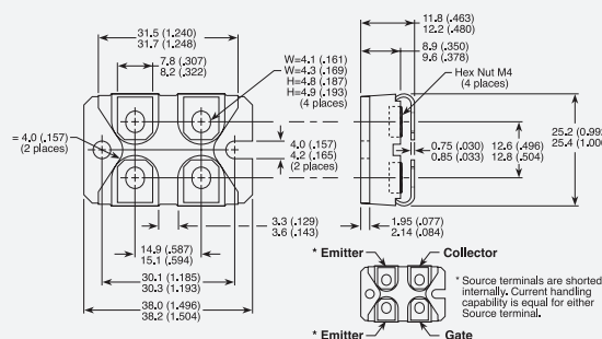
SOT-227
