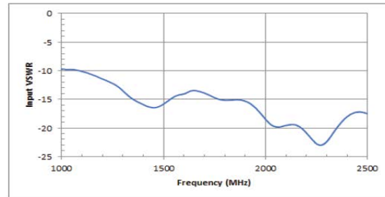
VSWR
