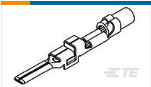
TE Part # 368086-1 090III NON SLD TAB(SQ 2.0)
