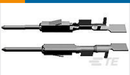
TE Part # 5-963716-1 MQS0,63 Sn tab LL unseal. 0,5-0,75
