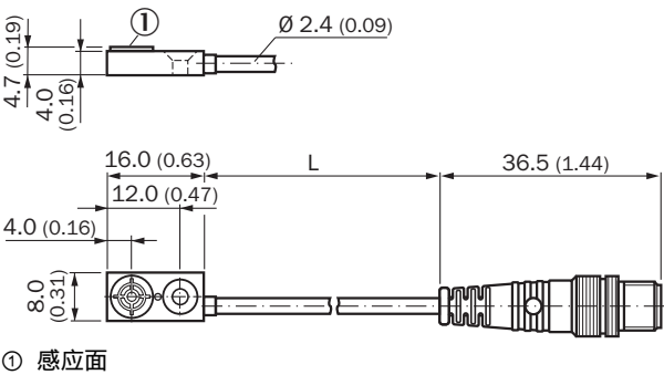
尺寸图 (尺寸单位: mm)
