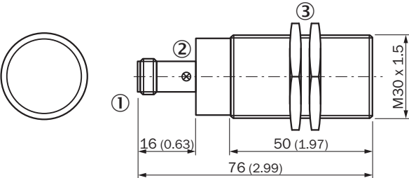
尺寸图 (尺寸单位: mm)
