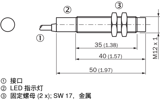
尺寸图 (尺寸单位: mm)
