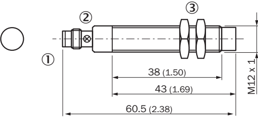
尺寸图 (尺寸单位: mm)
