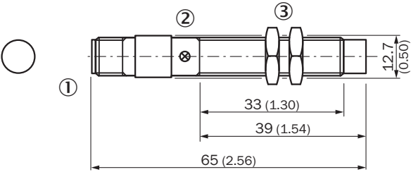
尺寸图 (尺寸单位: mm)
