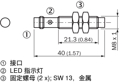
尺寸图 (尺寸单位: mm)
