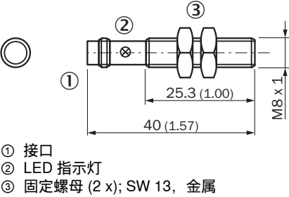
尺寸图 (尺寸单位: mm)
