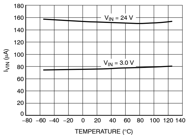
Figure 12. Vin Controller Current vs. Temperature (EN = HIGH)
