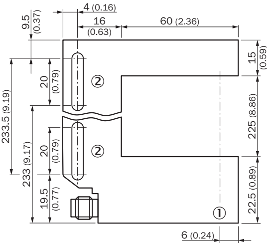
尺寸图 (尺寸单位: mm)
