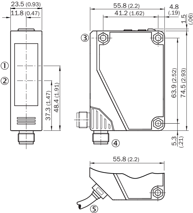
尺寸图 (尺寸单位: mm)
