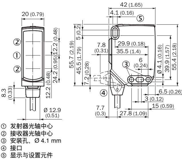
感测器尺寸圖
