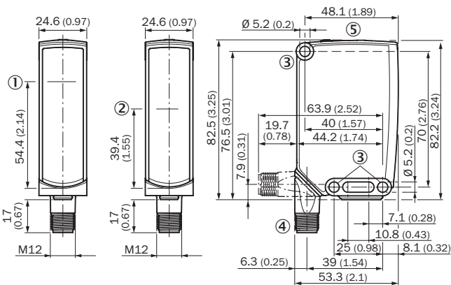
感測器尺寸圖
