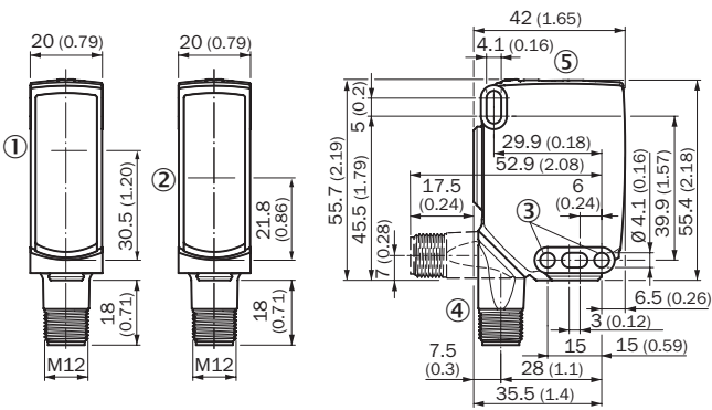
感測器尺寸圖
