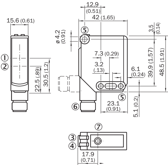
尺寸图 (尺寸单位: mm)
