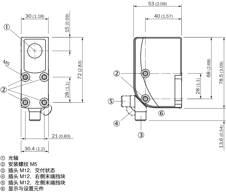
尺寸图 (尺寸单位: mm)
