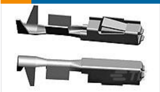
TE Part # 2141824-1 MQSQ,63 Sn rec LL unseal. 0,13-0,17
