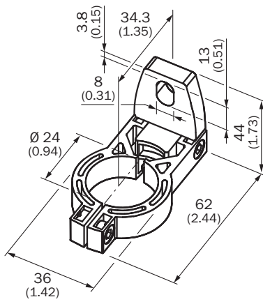
尺寸图 (尺寸单位: mm)
