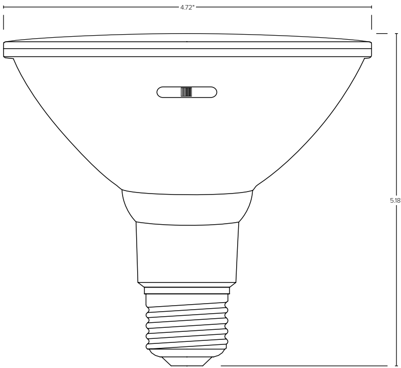
PAR38 13W
