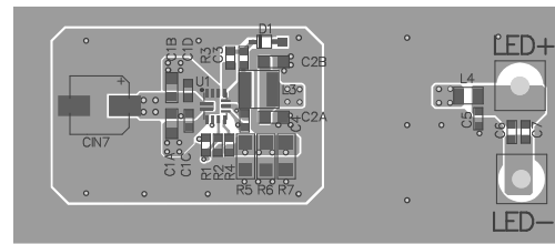
Top Layer
