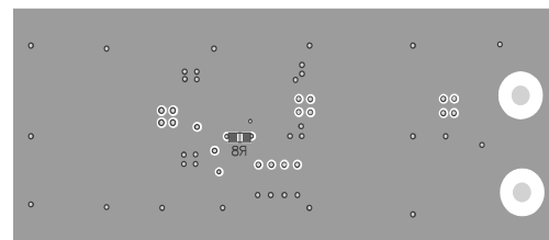
Bottom Layer
