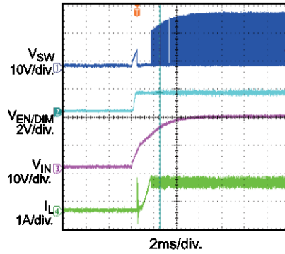
VIN Start-Up
