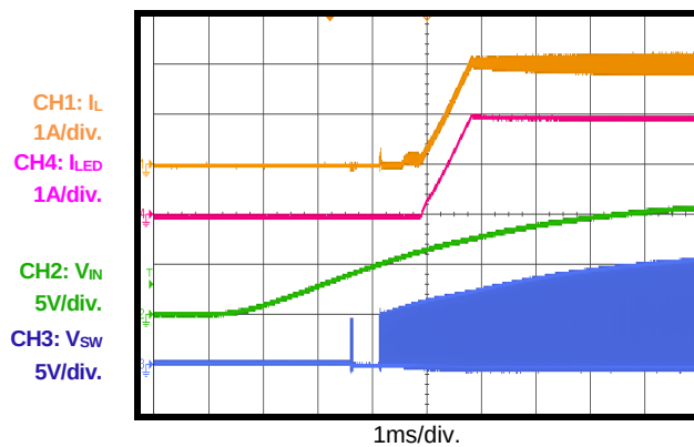
VIN Start-Up
