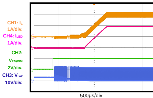
EN Start-Up
