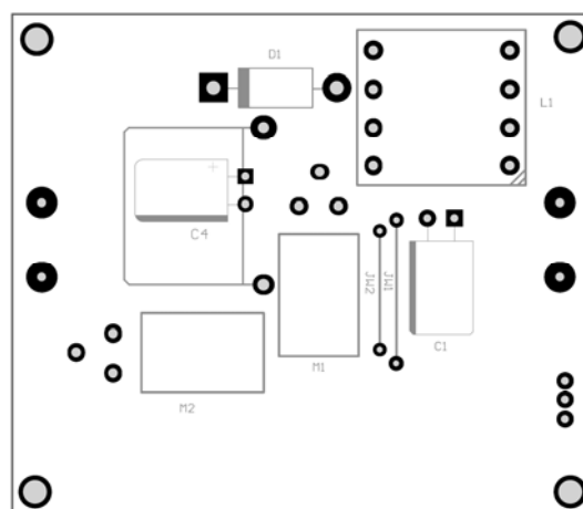
Figure 4—Bottom Layer
