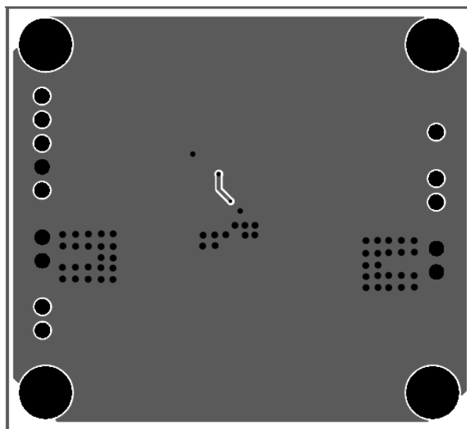
Figure 2—Bottom Layer
