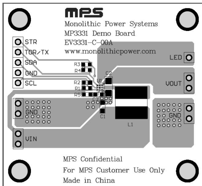
Figure 1—Top Layer
