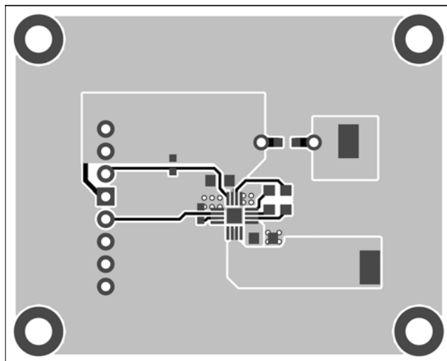
Figure 2—Top Layer
