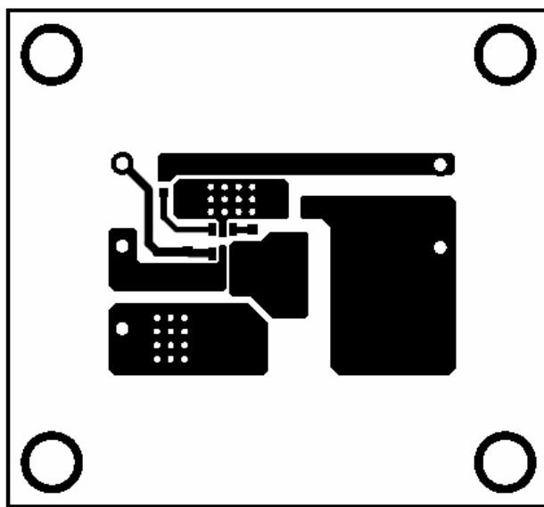
Figure 2—Top Layer
