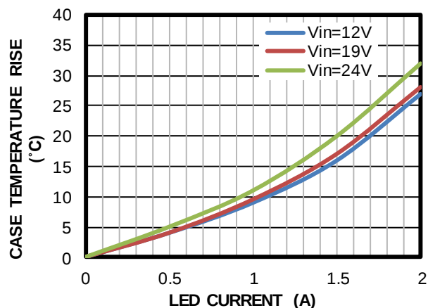
Thermal Test
