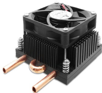
ATS-LQHS-84030-C1-R0 84.0 x 84.0 x 30.8mm Thermal Resistance: 0.05°C/W
