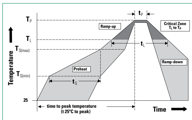
Soldering Parameters
