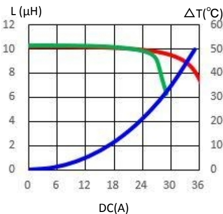
3. CDPQ2419NP-100LB-AL156
