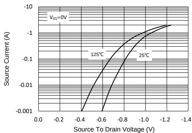
Fig.9 - I_S - V_{SD}
