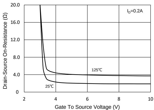
Fig.3 - R_{DS(ON)} - V_{GS}
