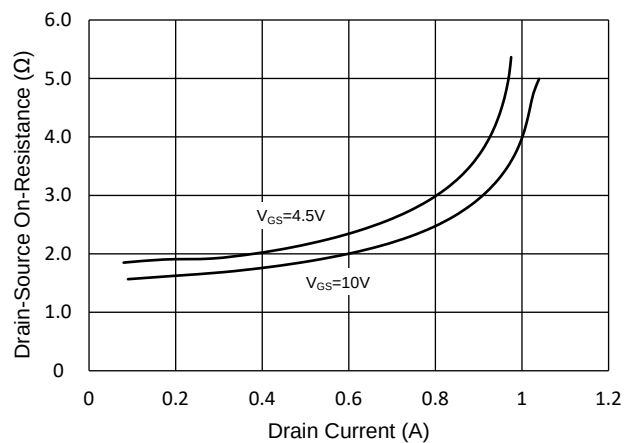
Fig.4 - R_{DS(ON)} - I_D
