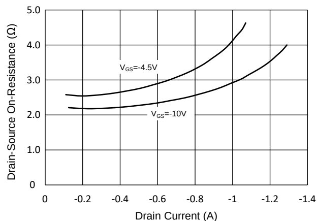
Fig.4 - R_{DS(ON)} - I_D
