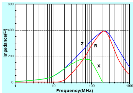
ACML-0805U-331
