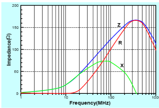
ACML-0805U-121
