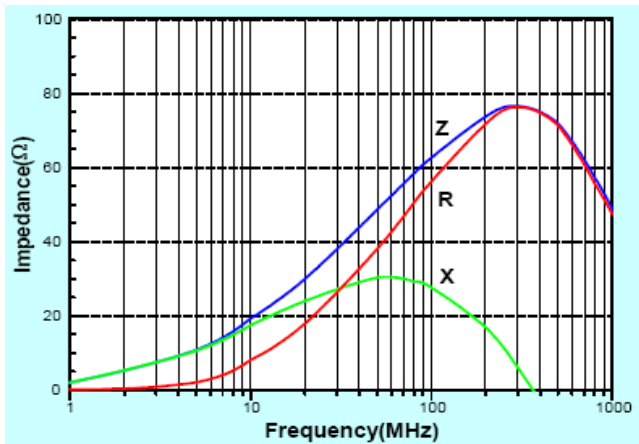
ACML-0805U-600
