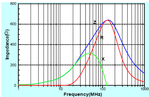
ACML-0805U-601
