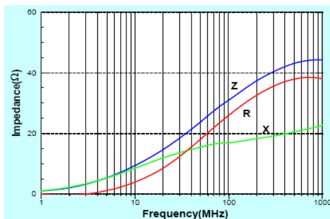
ACML-0805U-300
