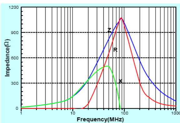
ACML-0805U-102
