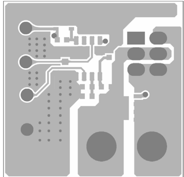
Figure 2—Top Layer
