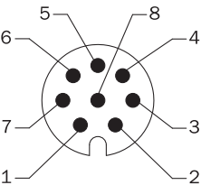
电缆/外壳上的设备插头 M12 视图
